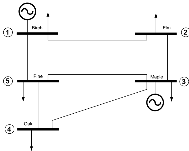
Figura – Diagrama unifilar do sistema 5 barras do Stevenson (pág.213)
